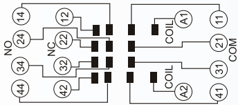
RÖLE SOKETİ SRN-08-SOK
