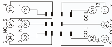
RÖLE SOKETİ SRN-11-SOK
