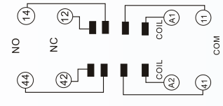
RÖLE SOKETİ SRN-14-SOK
