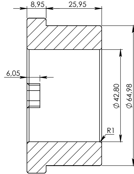
KESIT B-B
